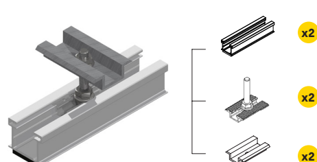
Tramo de perfil 150 mm con intermedia
