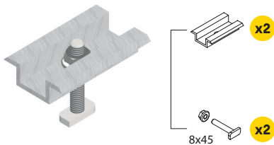
Grapa intermedia con tornillo
