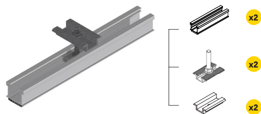
Tramo de perfil 300 mm con intermedia
